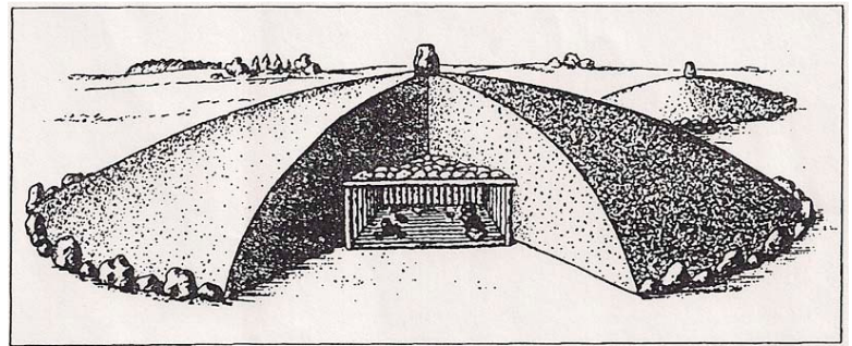
Innerer Aufbau eines hallstattzeitlichen Grabhügels.
